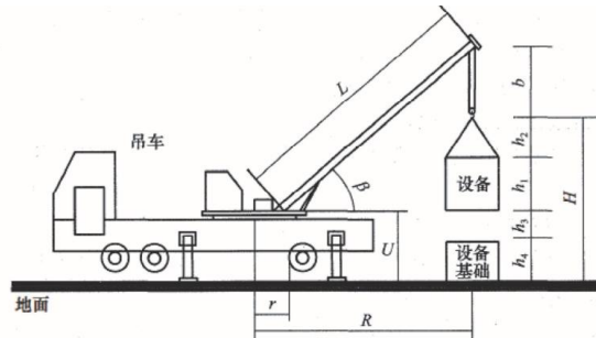
图 1H412021 起重机起吊高度计算简图
