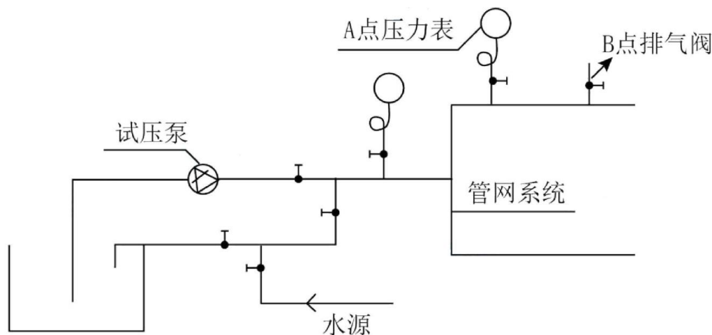
图3 临时试压系统示意图
